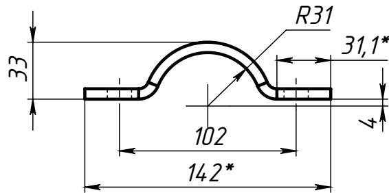
Поз.4 (Полухомут)
